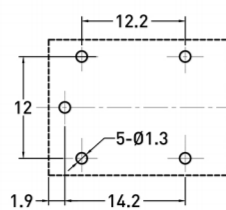
安装孔尺寸
