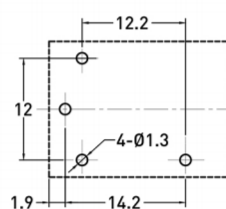
安装孔尺寸
